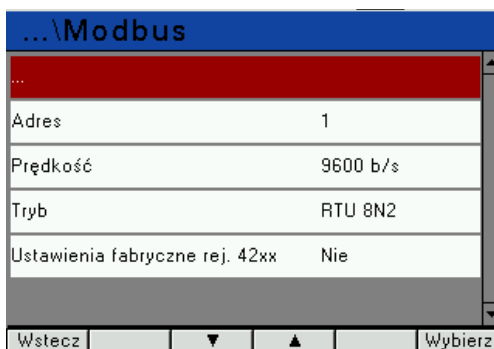
Rys.21. Ekran grupy Modbus
