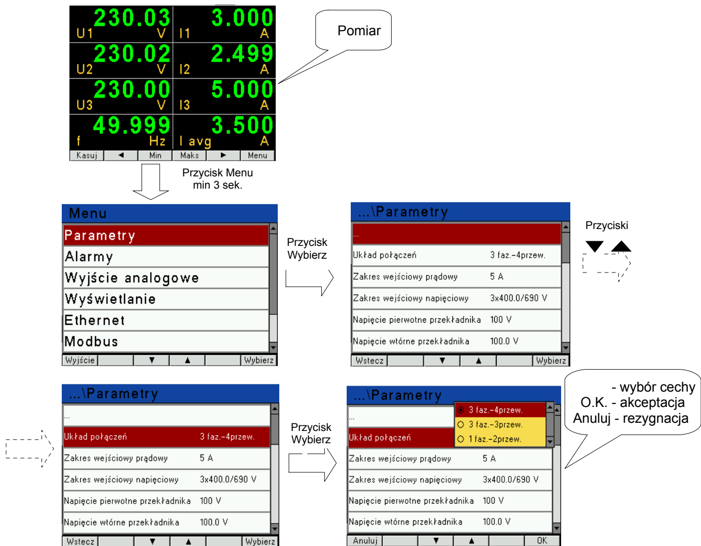
Rys.15. Ekran grupy Parametry
