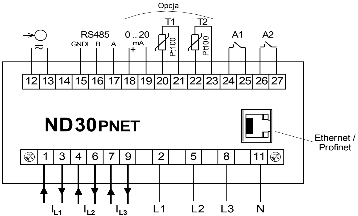
Rys.4a. Podłączenia miernika w wykonaniu z wejściami Pt100
