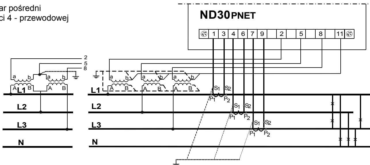
Rys.6. Podłączenia sygnałów wejściowych w sieci trójfazowej 4 – przewodowej
