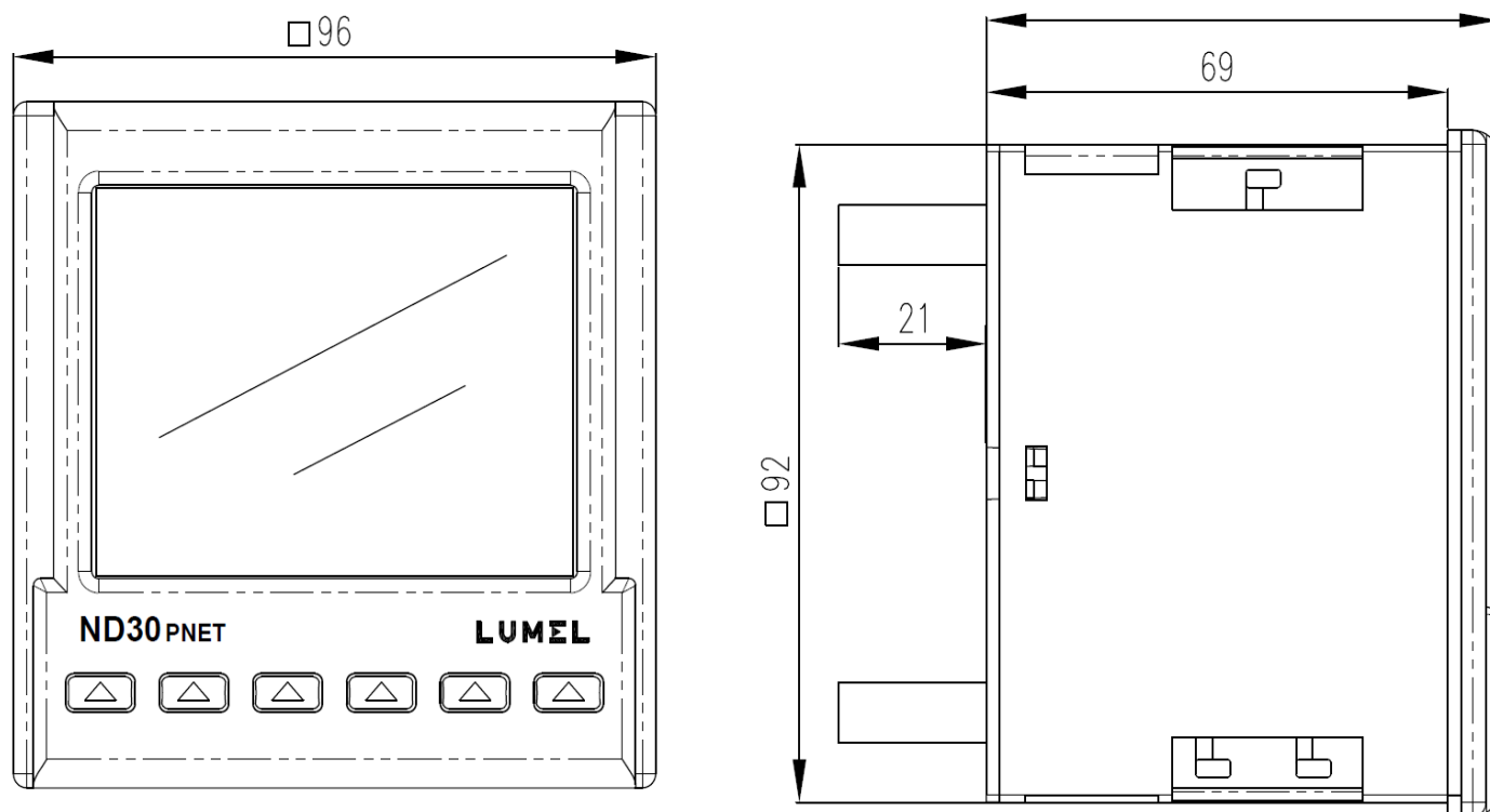
Rys.3. Rysunek gabarytowy miernika ND30PNET
