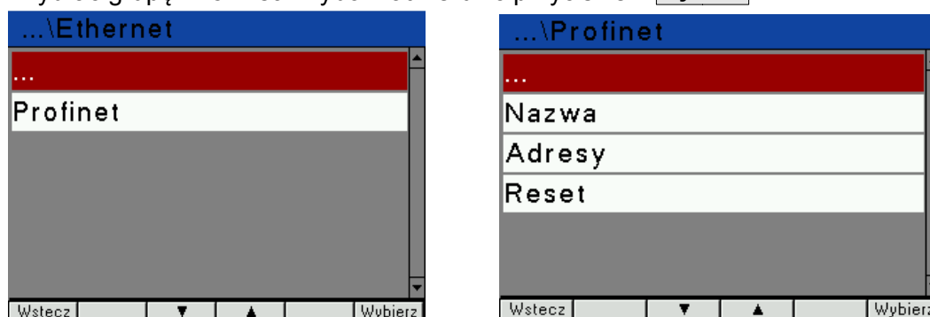
Rys.20. Ekrany grupy Ethernet / Profinet
