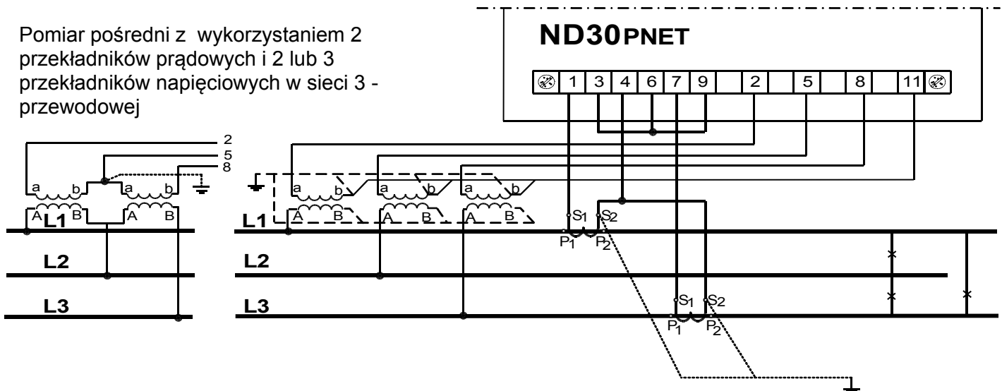
Rys.7. Podłączenia sygnałów wejściowych w sieci trójfazowej 3 – przewodowej
