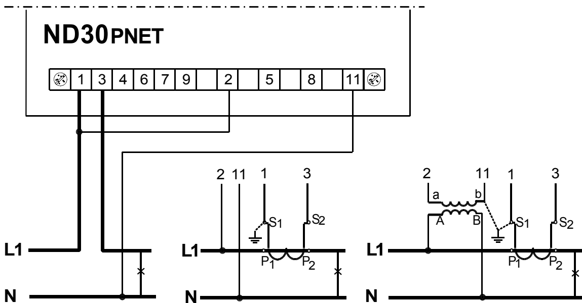
Rys.5. Pomiar bezpośredni, pośredni i pośredni w sieci 1-fazowej
