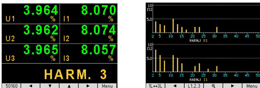
Rys.13. Ekran 11 i 12 - wizualizacja harmoniczných
