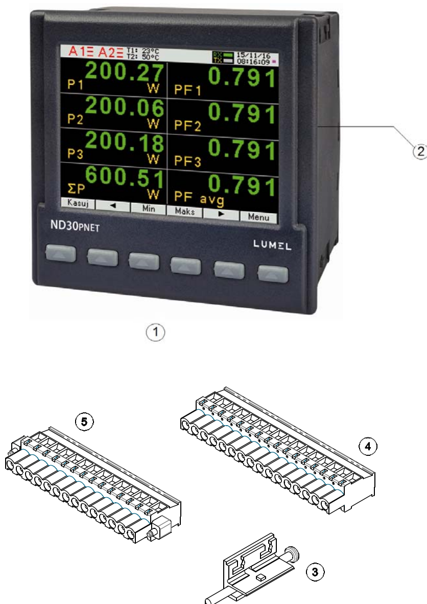
Rys.1. Zestaw miernika
