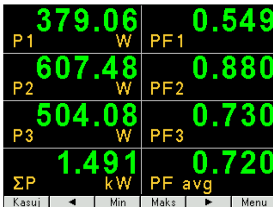
Rys.11. Ekran trybu pomiarowego miernika
