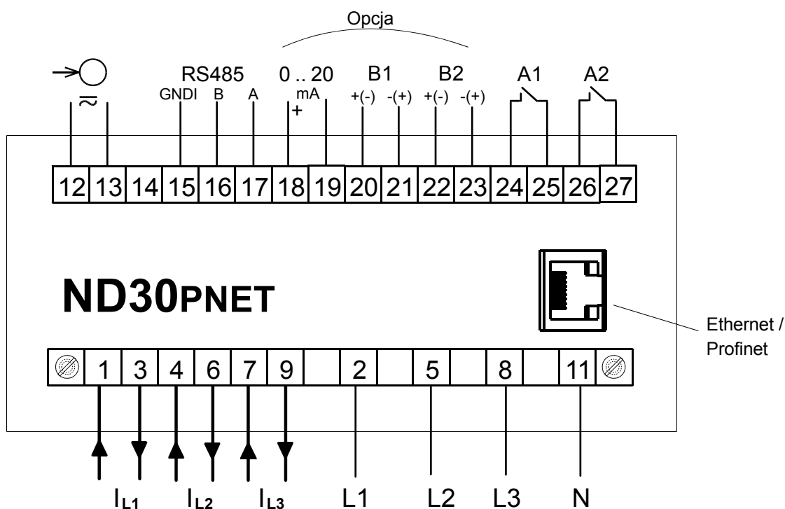
Rys.4. Podłączenia miernika w wykonaniu z wejściami binarnymi
